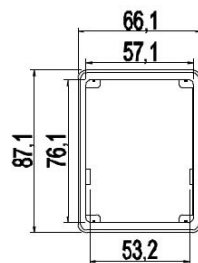
Рисунок 4-5. Монтажная платформа
