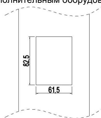
Установочный размер
