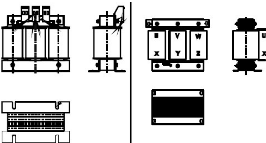
Входной реактор
