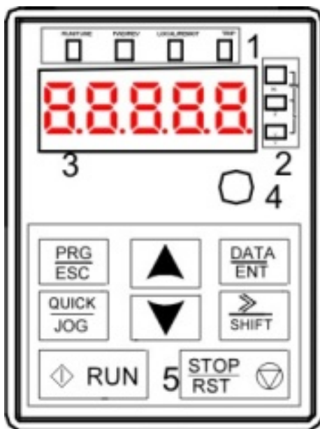
Рис.6-1 Панель управления
